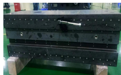
Torsion Test
